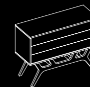
COMODA TWIGGY Medida: 120 x 45,5 x 90 cm Ref. TWG2201
